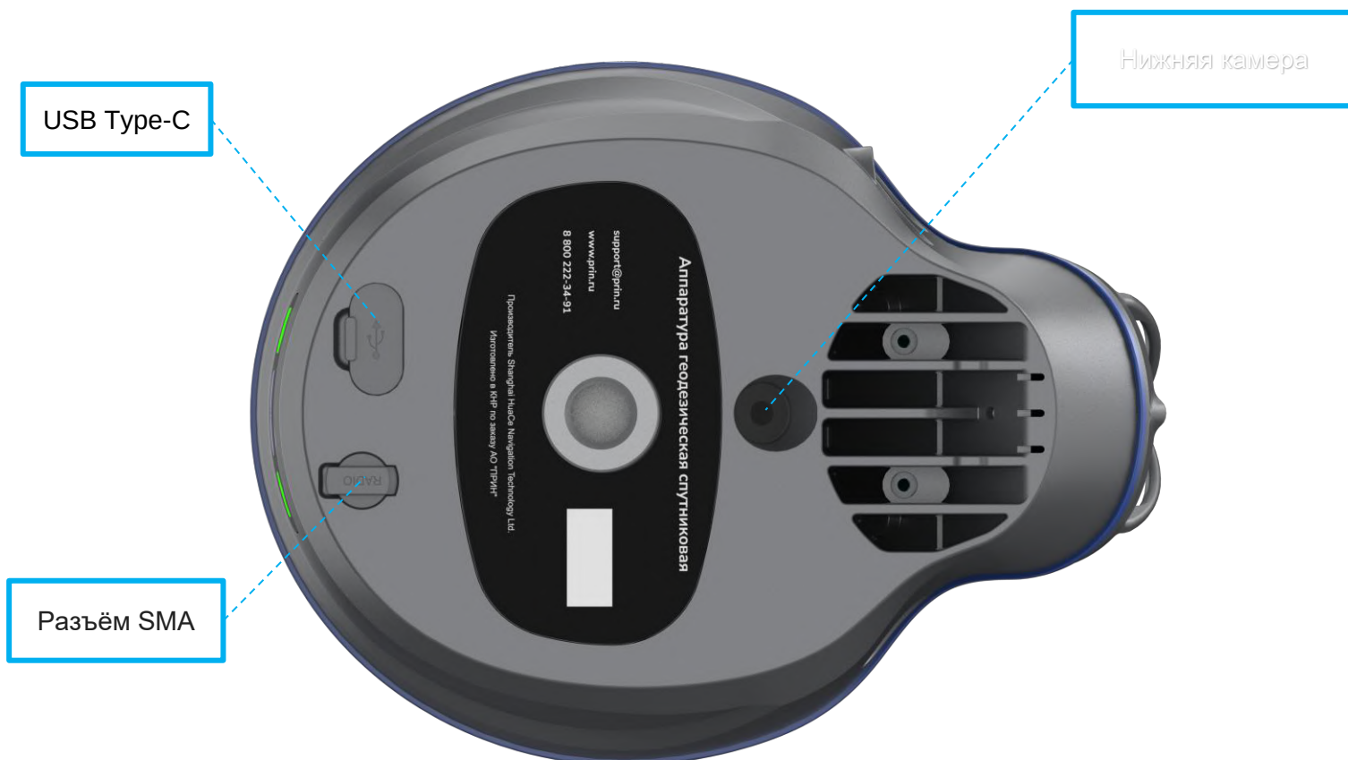
Рис. 1.2 Нижняя часть PrinCe i95XR
