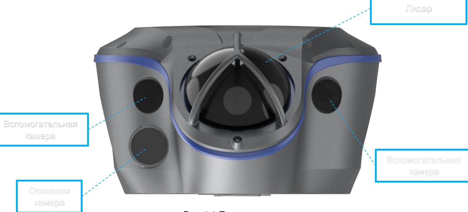
Рис. 1.1 Передняя панель
