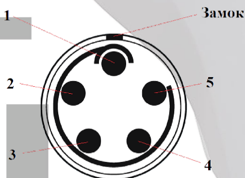
Распиновка порта LEMO (5-pin) приемника AlphaGEO A8 Plus:
